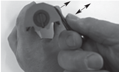
Kammerstengel nach unten bewegen und durch etwas hin- und her bewegen entnehmen.
